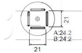
A1182B BQFP 24 x 24
